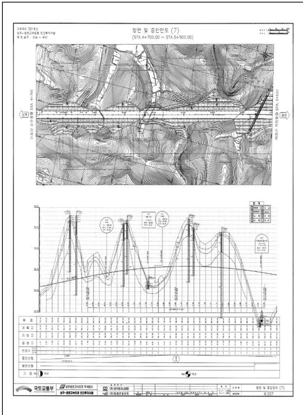
【그림 46.1.4】 평면도
